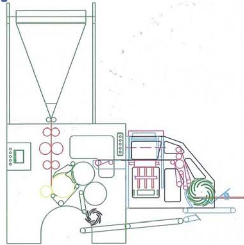
PRESS TECH 固定尺寸、有销折页机
