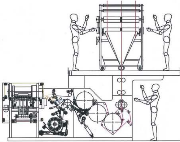
FOLDEX 可变尺寸、无销折页机
